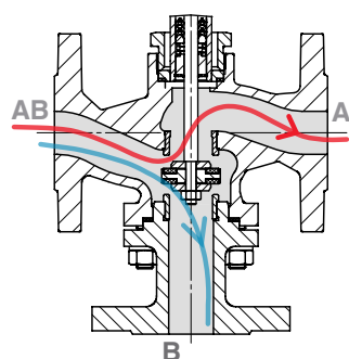
GEMÜ 312 Distribution
