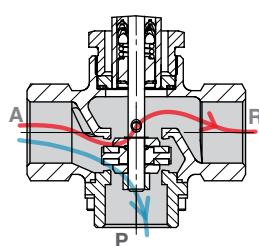
GEMÜ 314 Distribution
